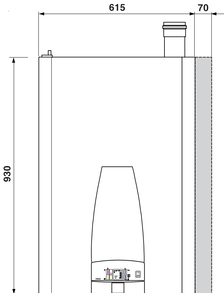
HOMLOKNÉZET
